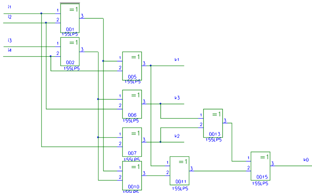
Рисунок 4. Схема формирования контрольных разрядов модифицированного кода Хемминга
