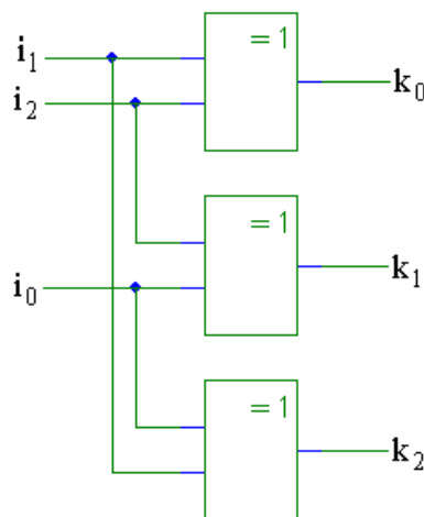
Рисунок 2. Схема формирования контрольных разрядов инверсного кода
