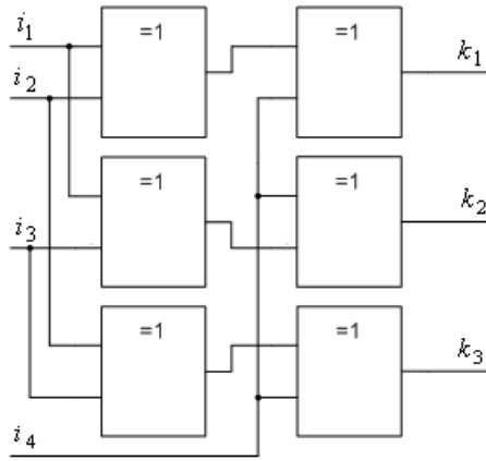
Рисунок 3. Схема формирования контрольных разрядов кода Хемминга
